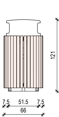
КАНТА ЗА ОТПАТКЕ - БОЧНИ ИЗГЛЕД 1:25
