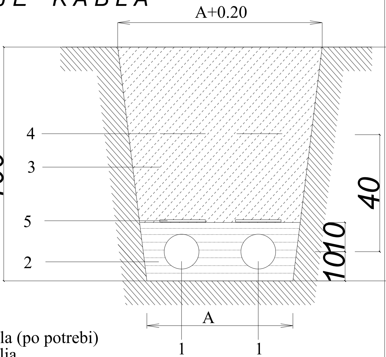
NA REGULISANOM TERENU
