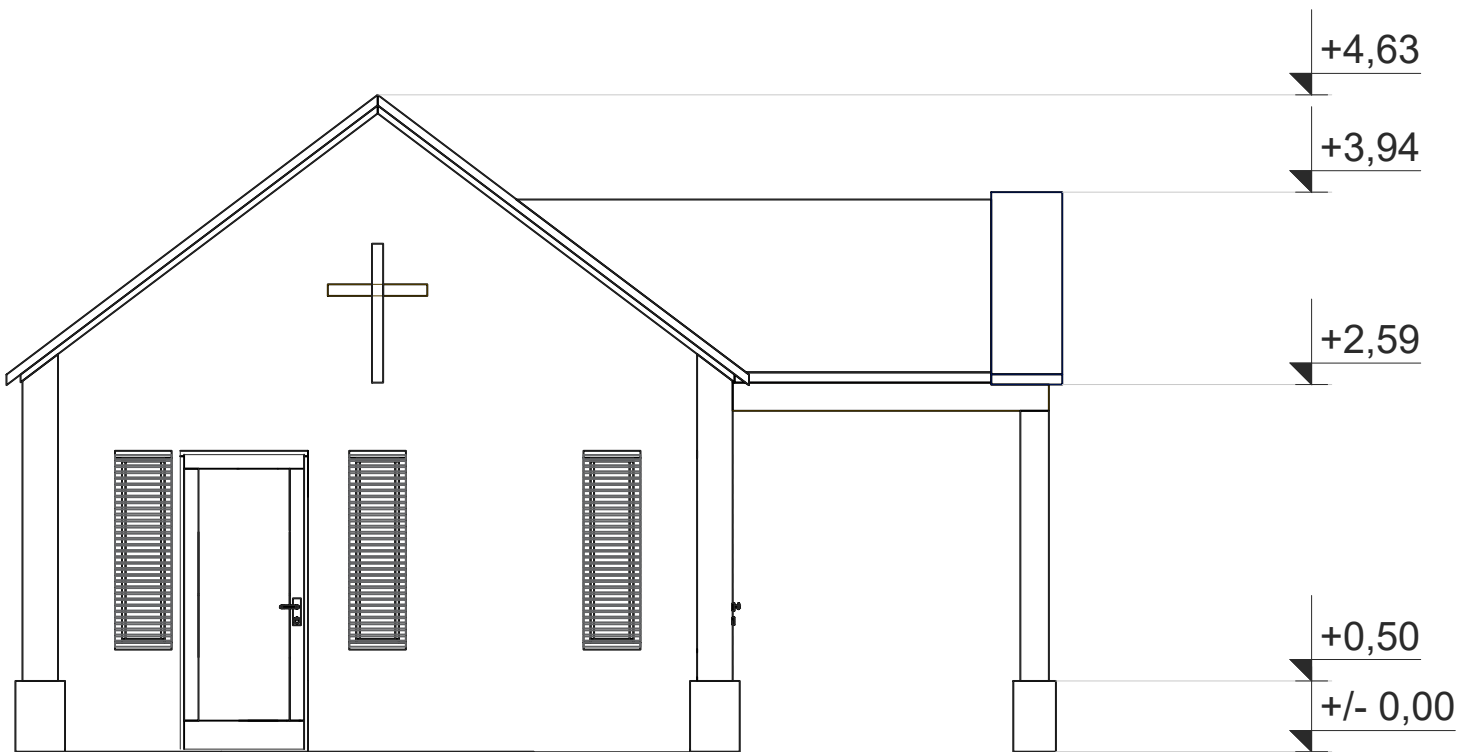
ЗАПАДНА ФАСАДА
