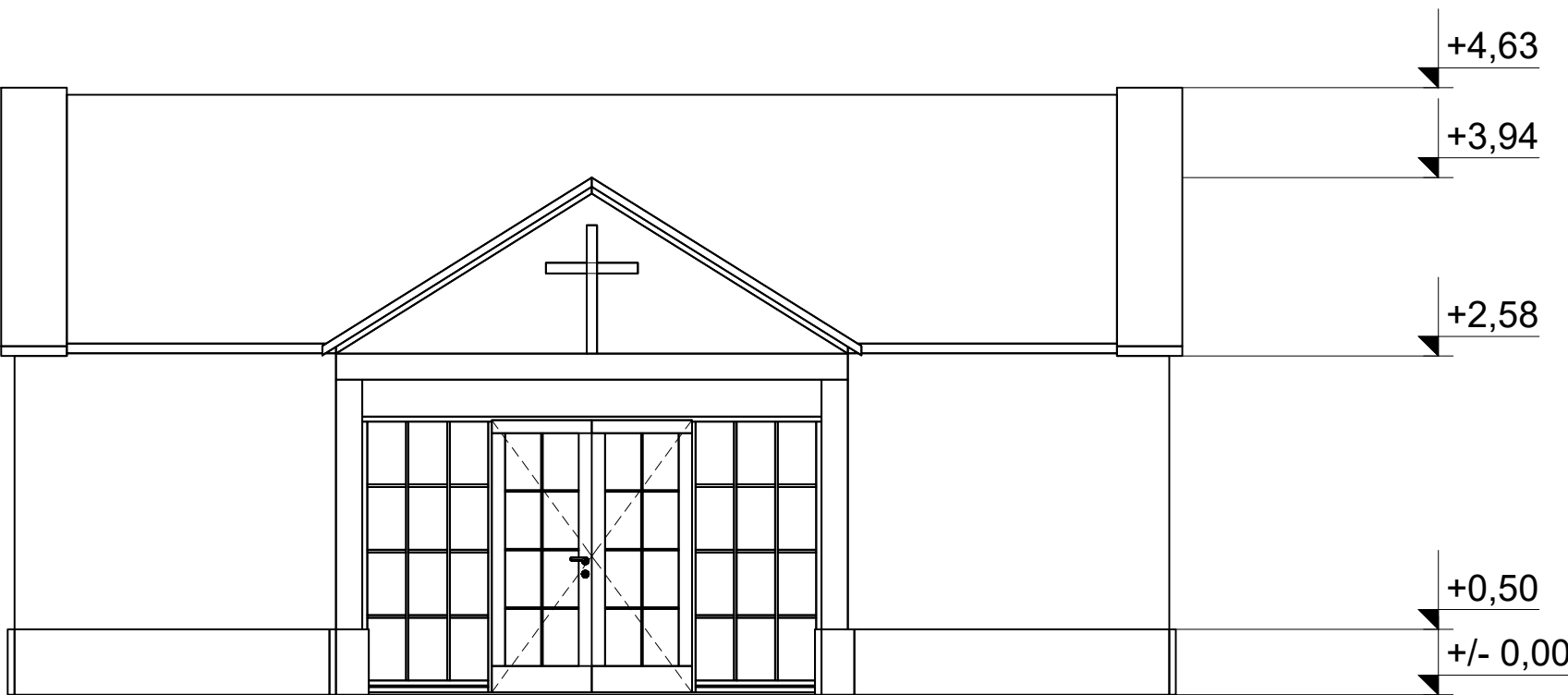
ЈУЖНА ФАСАДА
