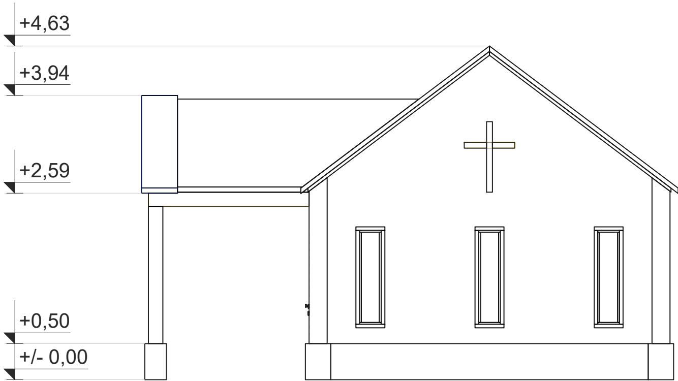
ЗАПАДНА ФАСАДА
