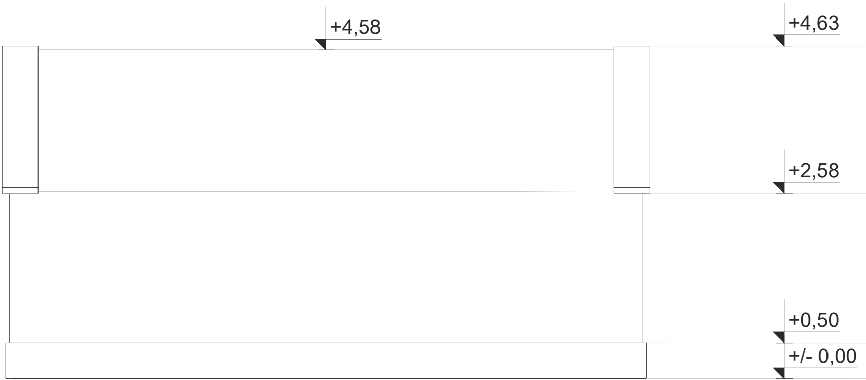
ЈУЖНА ФАСАДА
