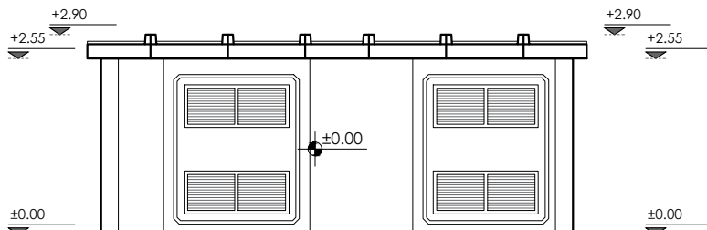
ZAPADNA FASADA
