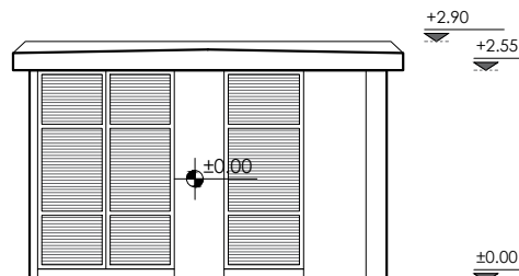
JUŽNA FASADA
