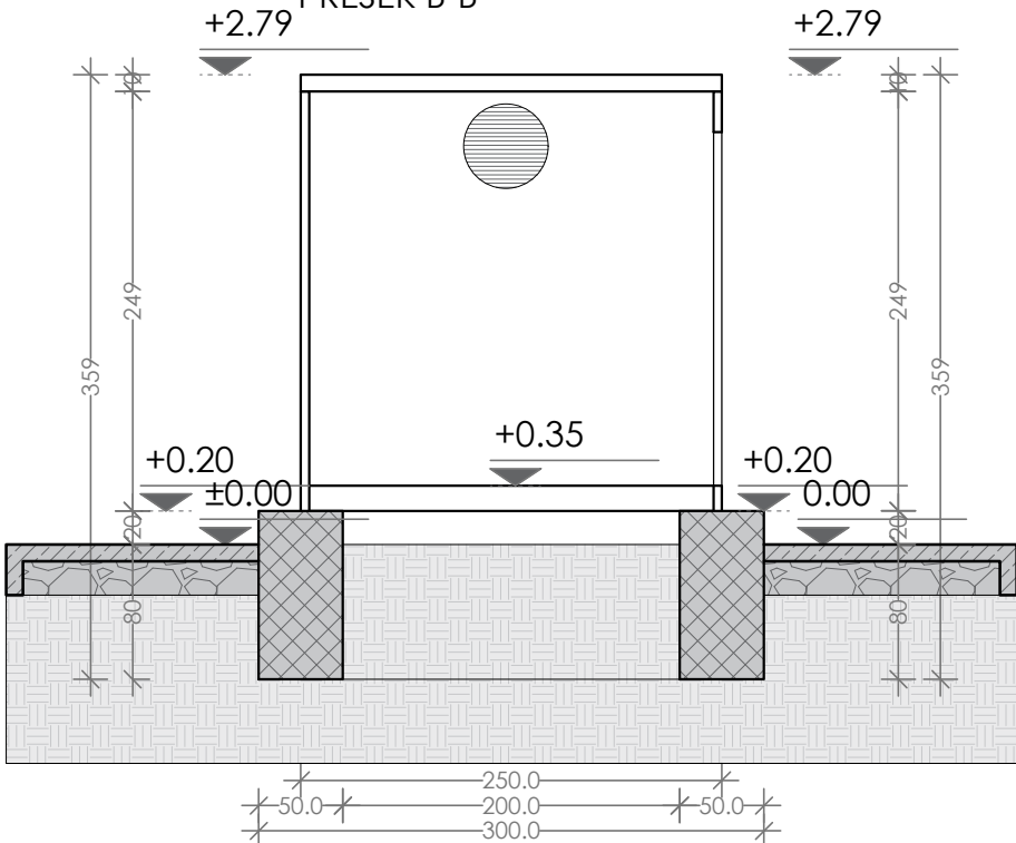
PRESEK B-B
