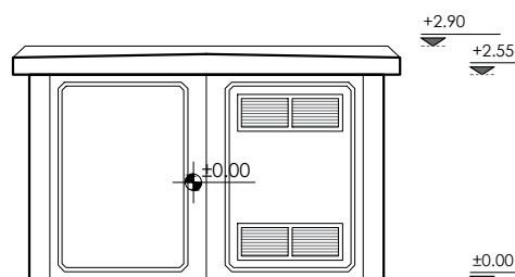
SEVERNA FASADA
