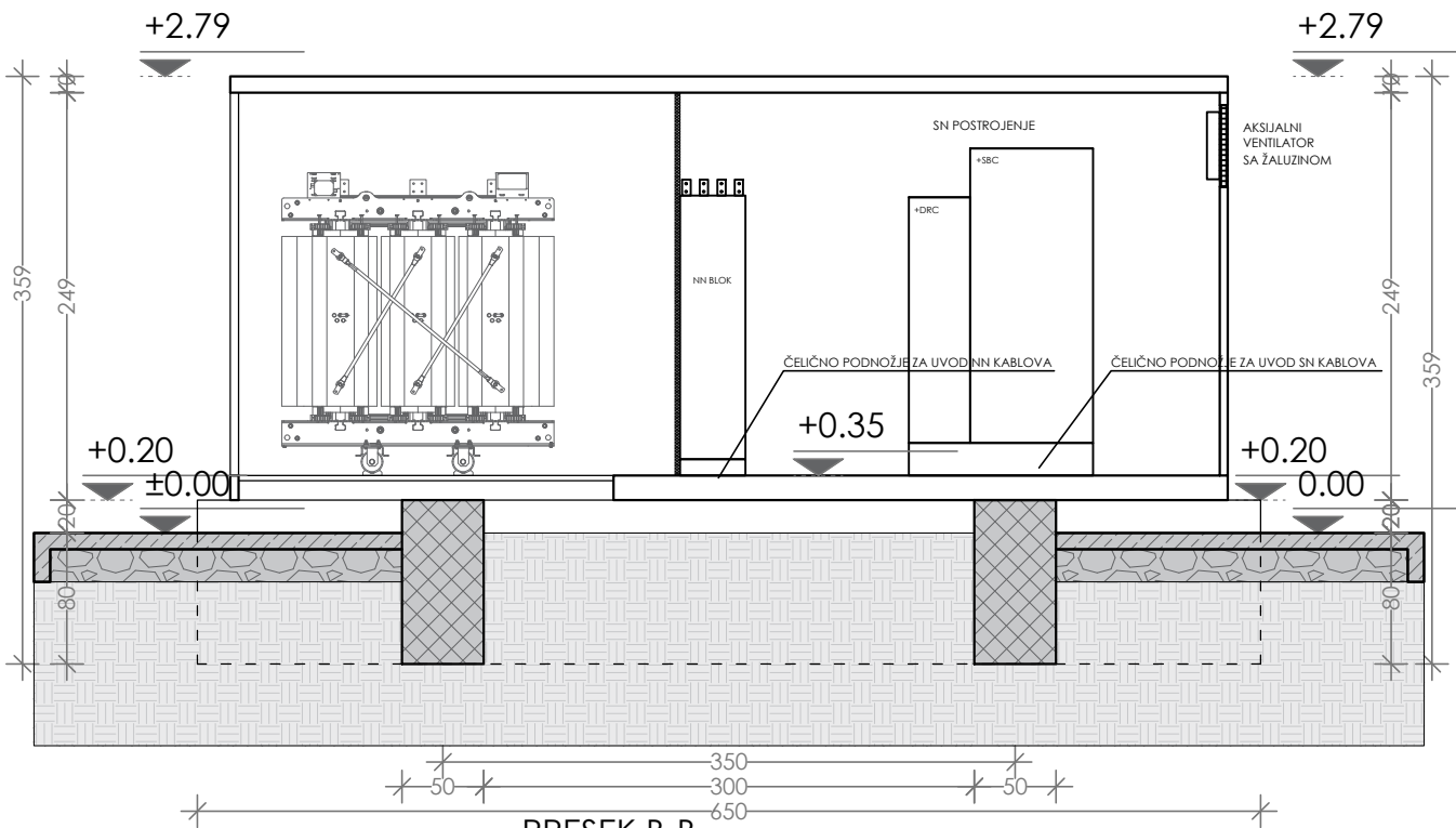
PRESEK B-B
