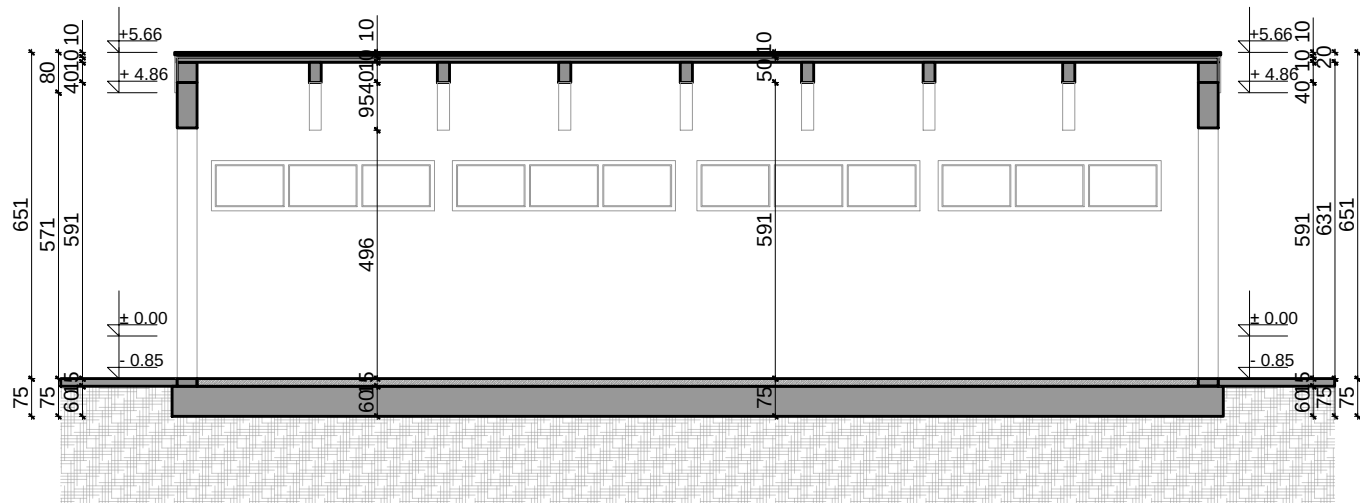
PRESEK 4-4
