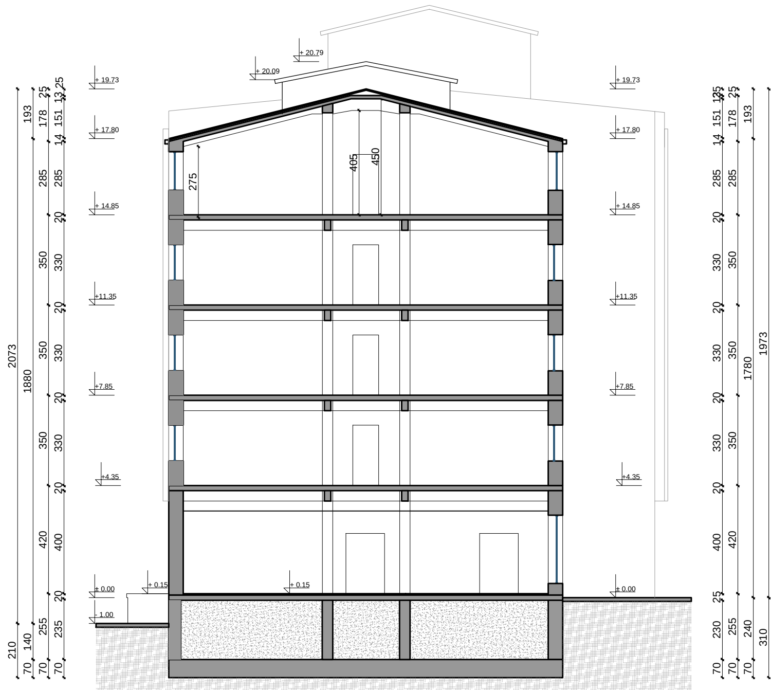
PRESEK 2-2
