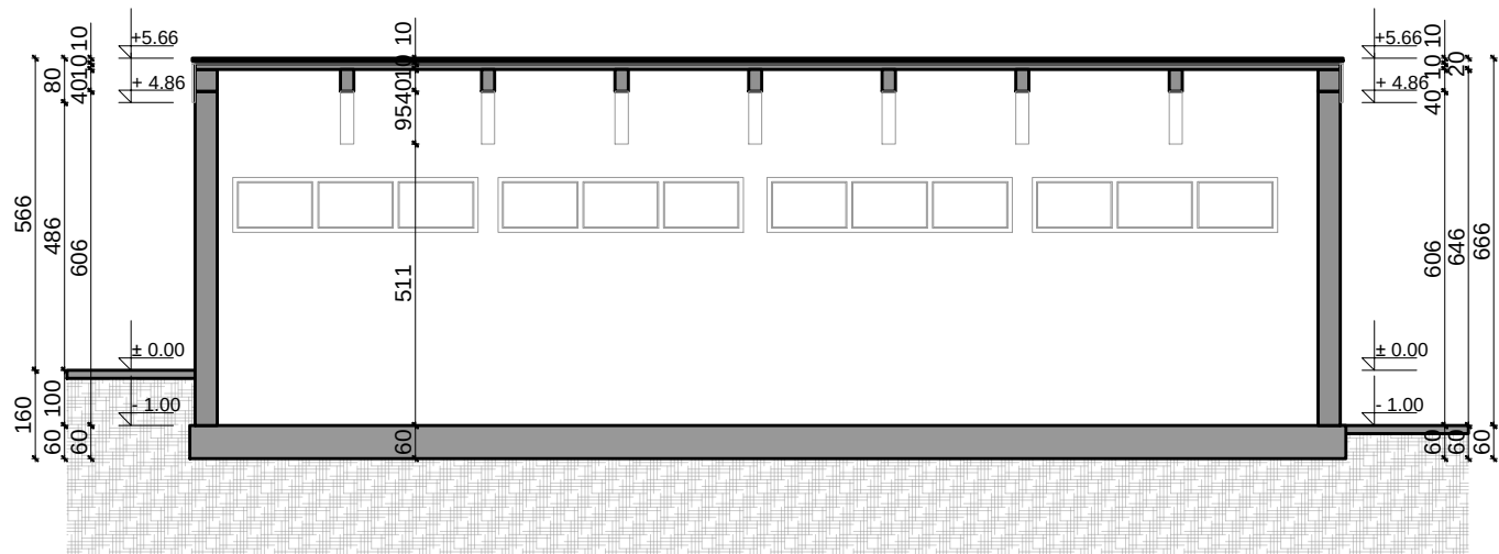
PRESEK 3-3
