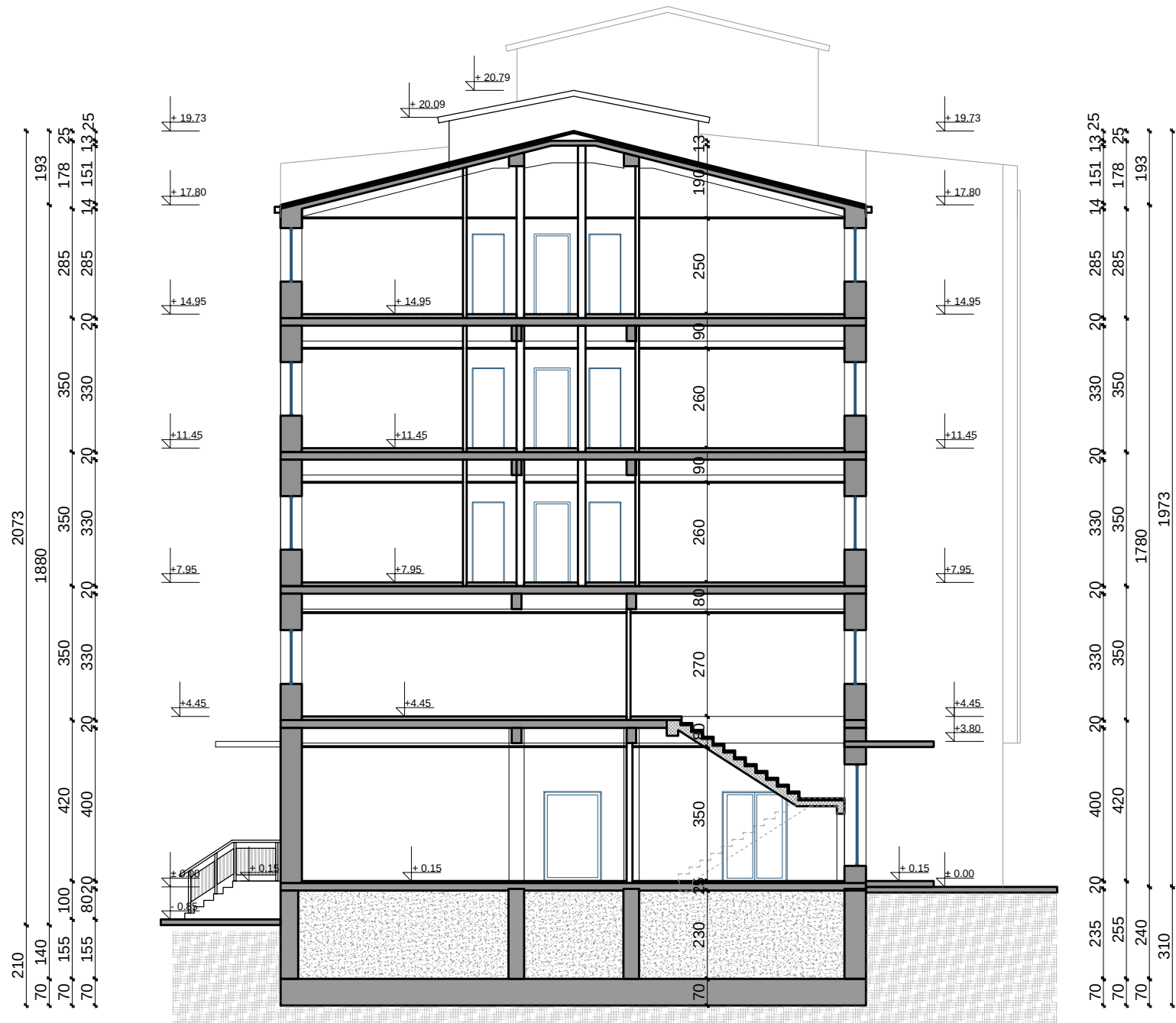
PRESEK 3-3
